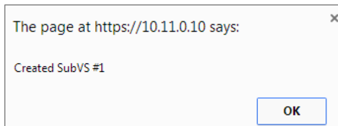
図 3-20: SubVS の作成
