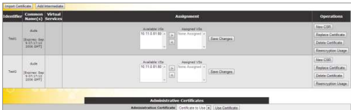
図 8-1: SSL 証明書
