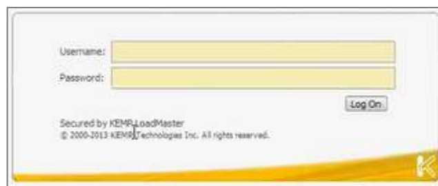
図 3-16: Blank Form
