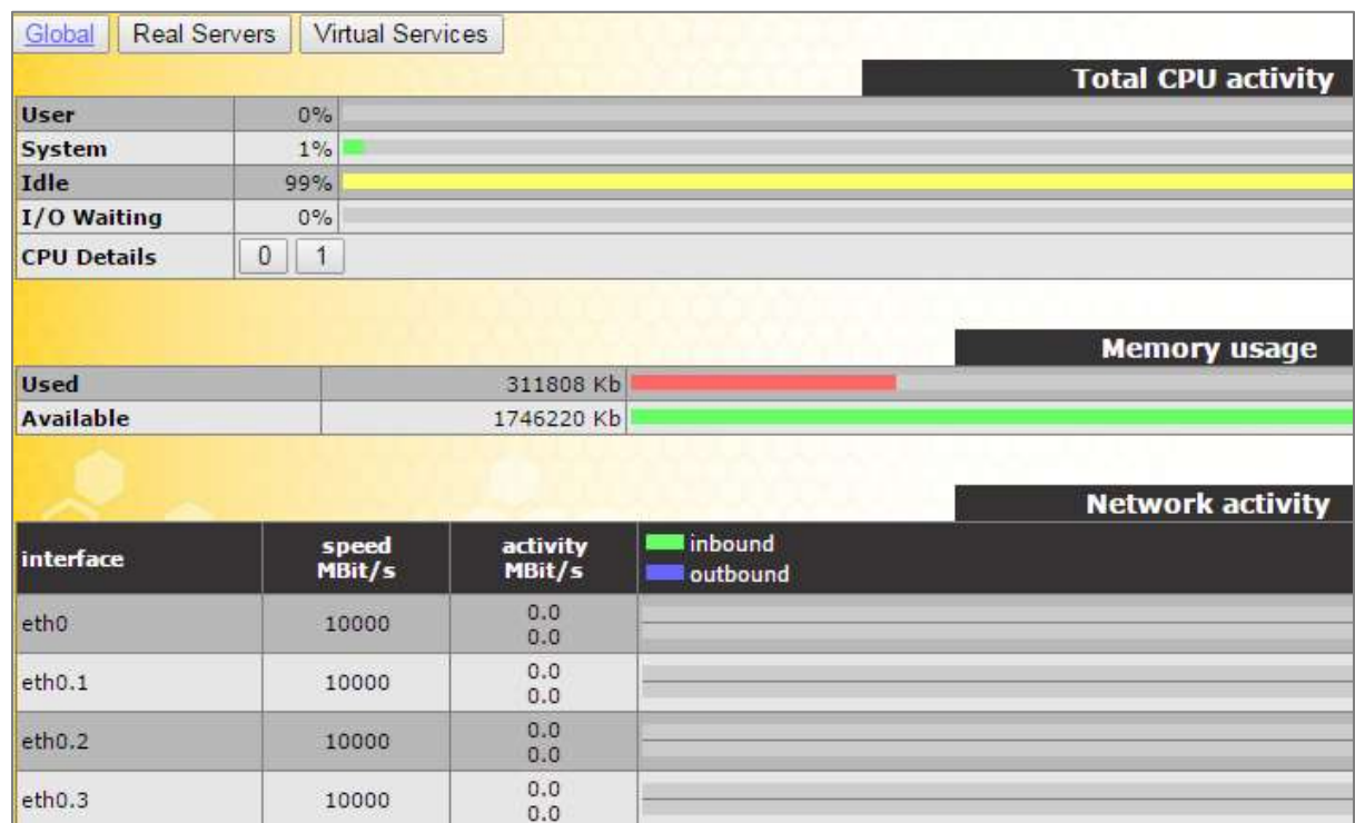
図 5-1: 統計
