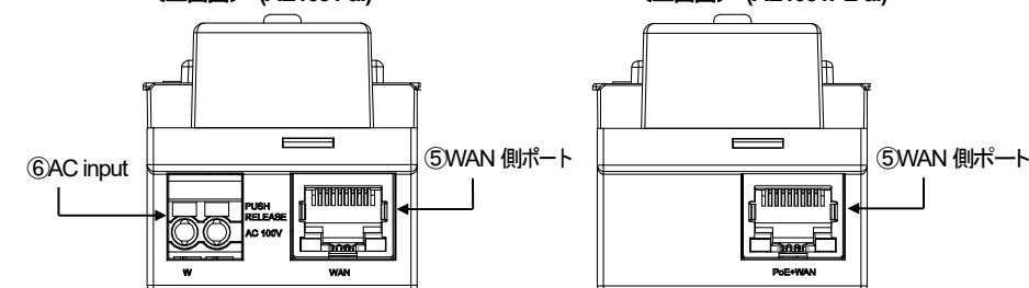
<上面図> (AE1031-ai)
