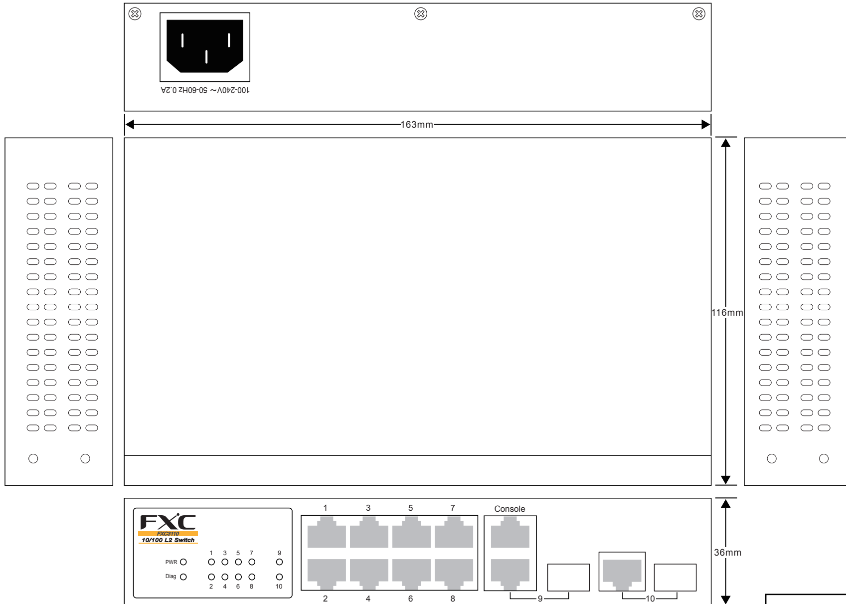
FXC3110外觀図
