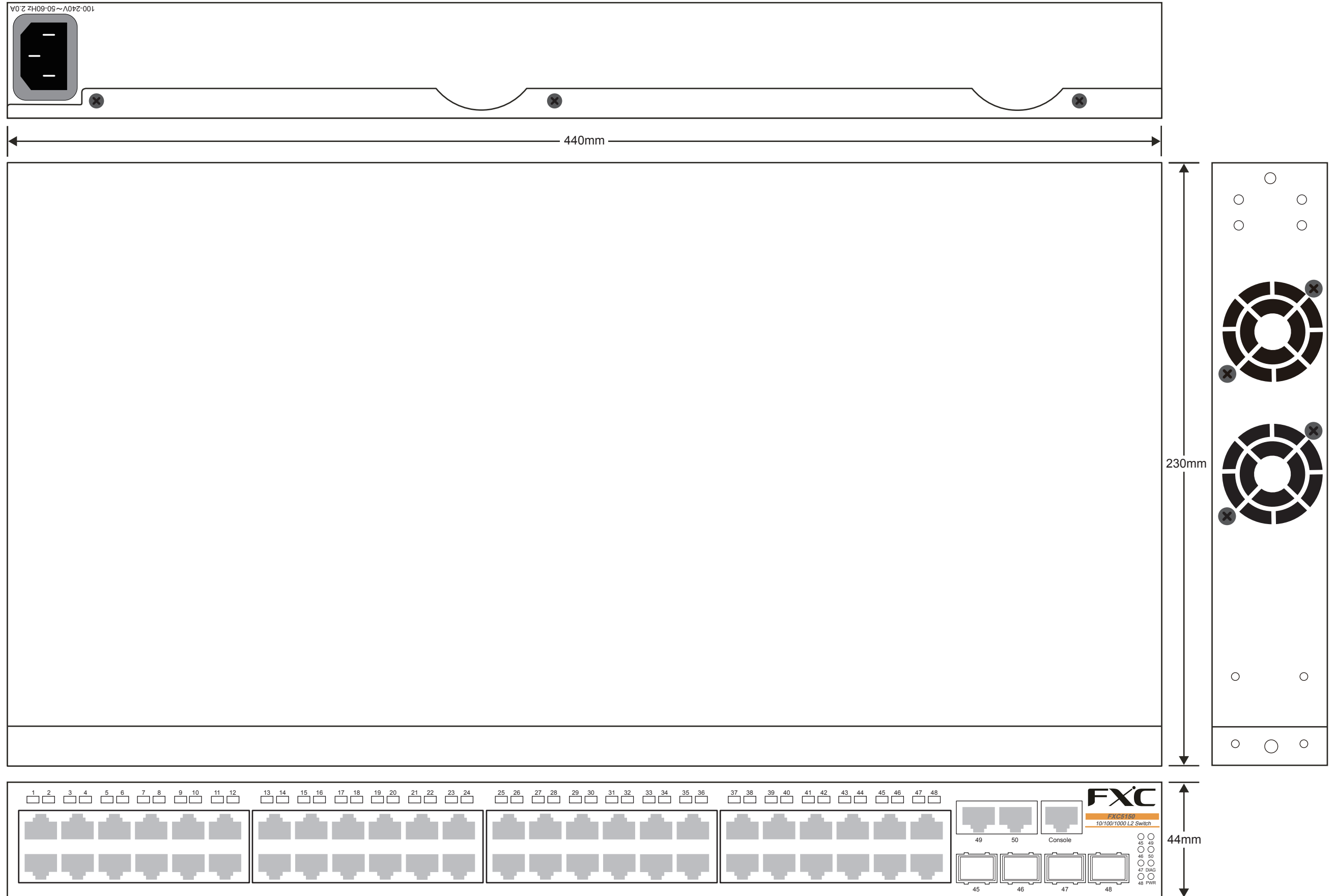
FXC5150外觀圖
