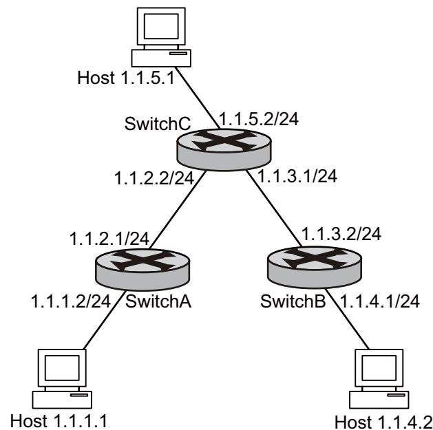
図 19 スタティックルート設定例のネットワーク構成図
