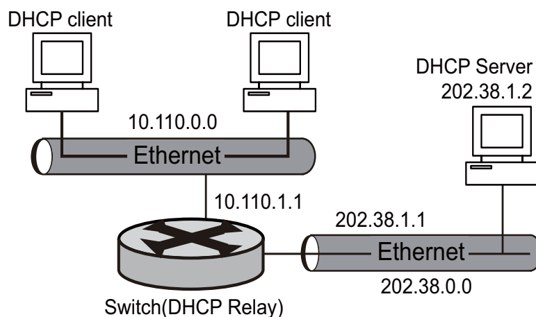
図 37 DHCP リレーを設定しているネットワーク構成図
