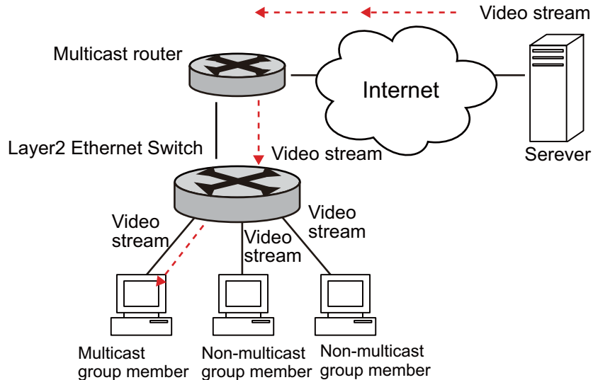
図 29 IGMP スヌーピングが稼働時のマルチキャストパケットフォワーディング
