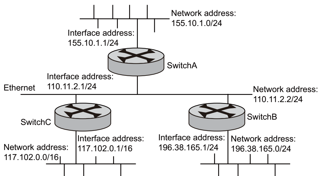
図 20 RIP を設定したネットワーク
