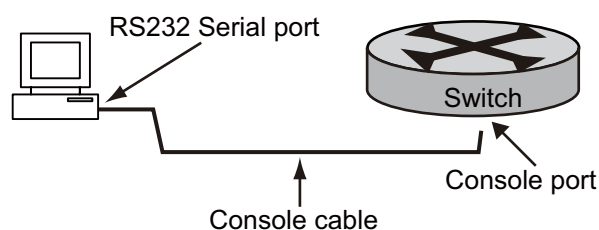
図 1 コンソールポートを介したローカル設定環境のセットアップ
