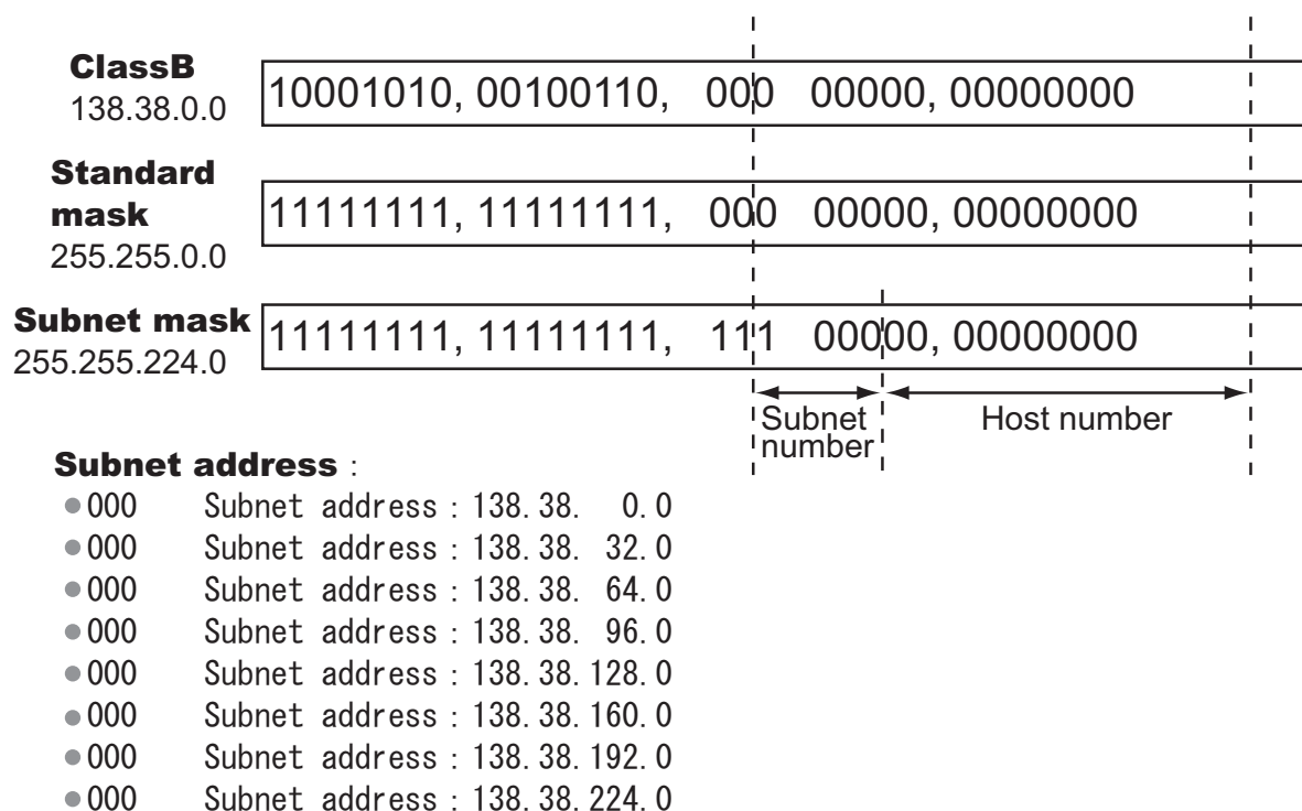
図 15 IP アドレスの分割によるサブネット
