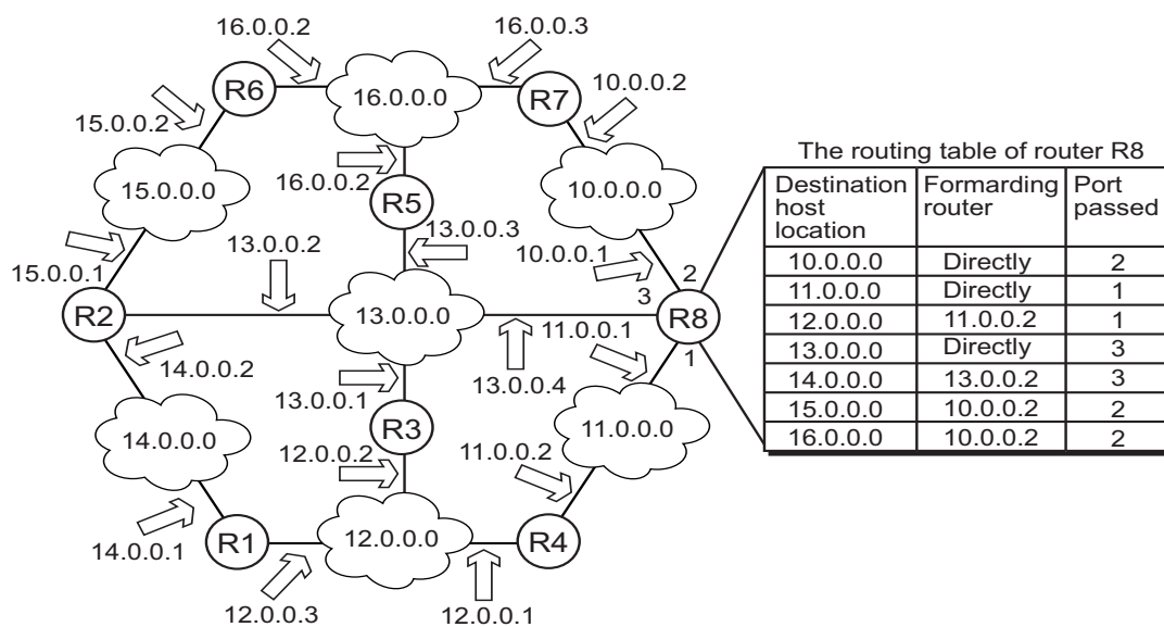
図 18 ルーティングテーブル
