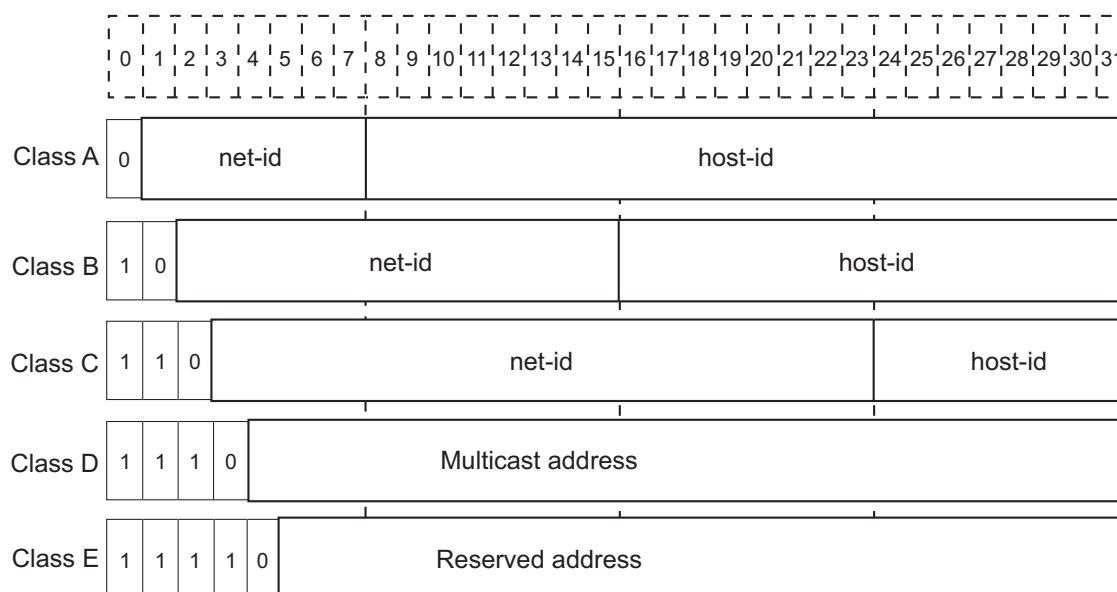
図 14 IP アドレスの 5 つのクラス
