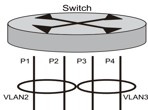
図 8 VLAN 構築例
