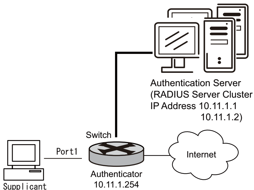
図 35 サプリカントで AAA を実行するよう IEEE 802.1x と RADIUS を有効化
