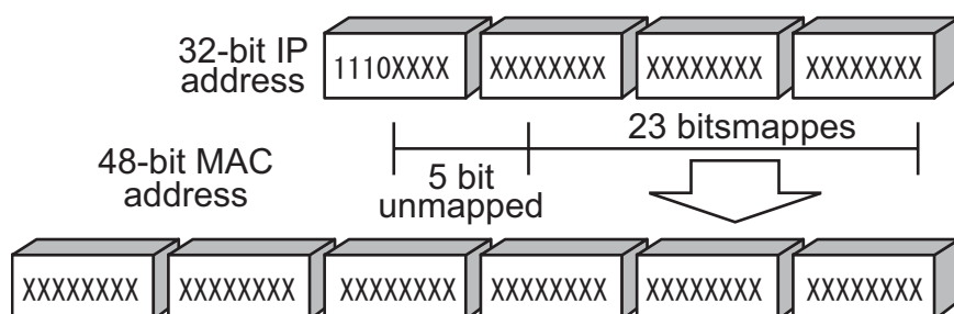
図 26 マルチキャスト IP アドレスとイーサネット MAC アドレスのマッピング
