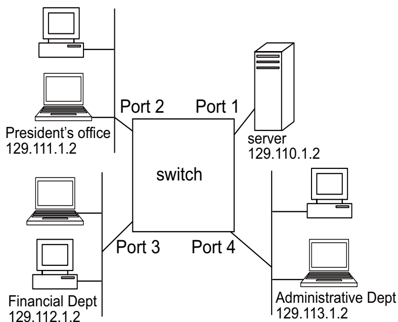
図 33 より高度な ACL を設定したネットワーク
