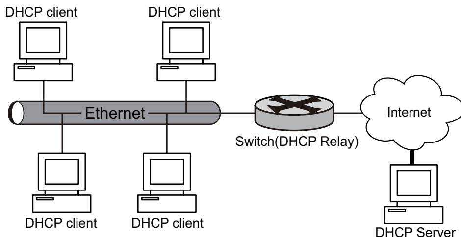
図 36 DHCP リレーの典型的なアプリケーション
