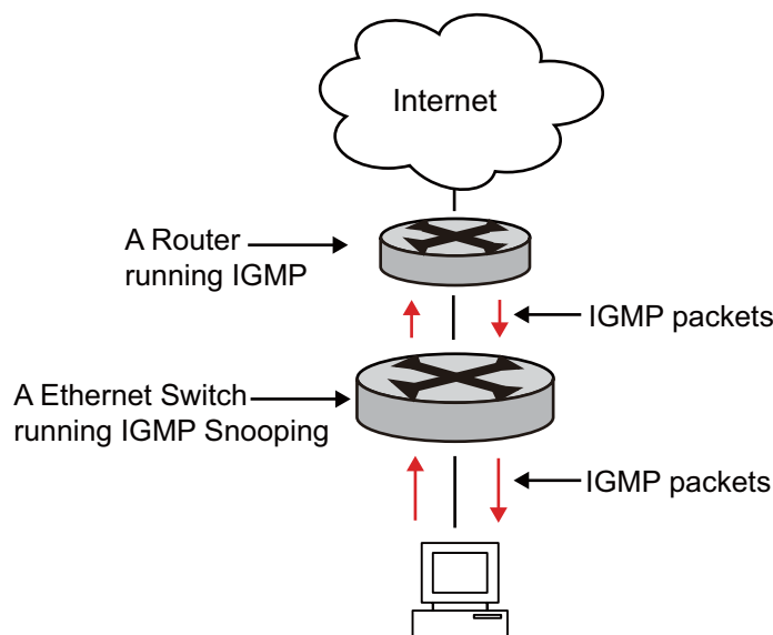
図 30 図 14-8 IGMP スヌーピングの実装
