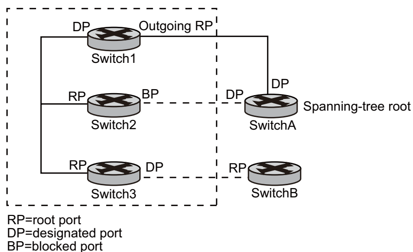
図 10 スタック構成のスイッチにおけるスパニングツリーのポートの状態
