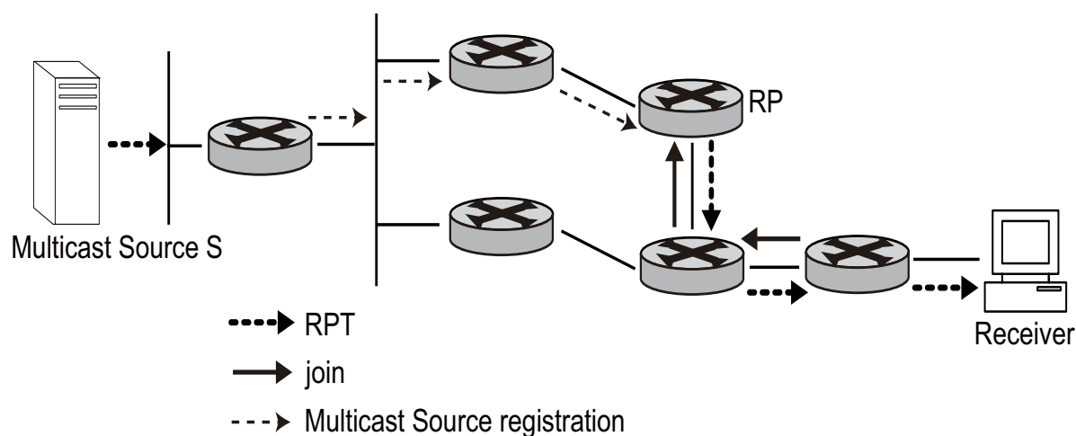
図 32 RPT 概略図
