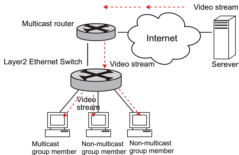
図 28 IGMP スヌーピングが無効の場合のマルチキャストパケットフォワーディング
