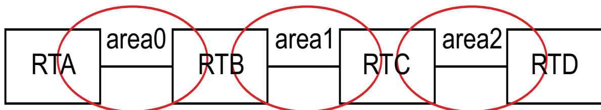
図 22 OSPF のエリア
