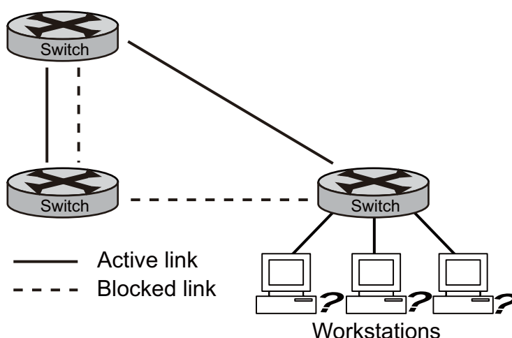
図 13 スパニングツリーと冗長接続性
