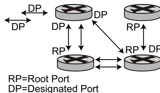
図 12 スパニングツリーのトポロジ
