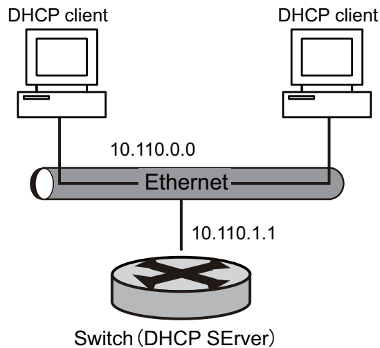
図 38 DHCP サーバを設定しているネットワーク構成図
