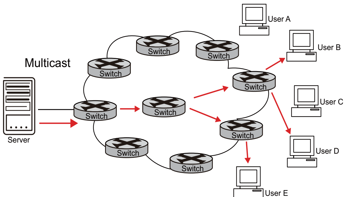
図 25 マルチキャストモードでのデータ転送
