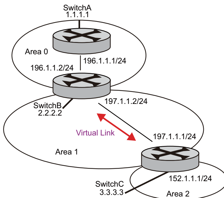
図 21 OSPF 仮想リンクを設定しているネットワーク
