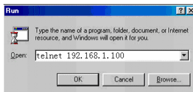
図 6 Telnet の実行
