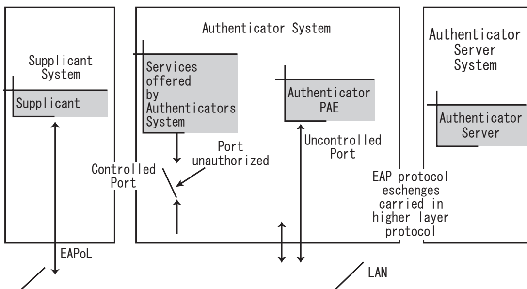
図 34 IEEE 802.1x システムアーキテクチャ
