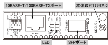
<前面図> LE2841-1F
