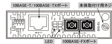
<前面図> LE2842-02/15
