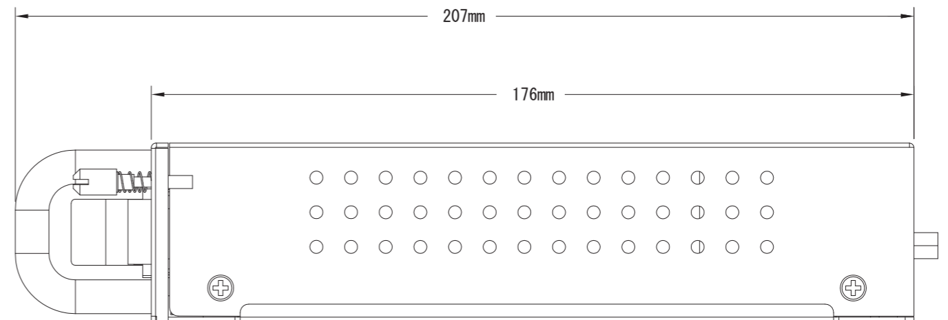
LEX1910-45外觀圖
