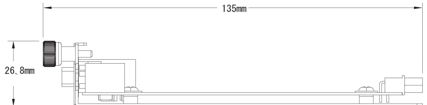
LEX1930-00外觀圖
