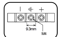
入力端子台イメージ図
