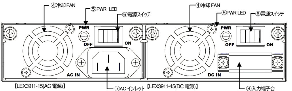
LEX3004 背面のイメージ図(LEX3911-45、LEX3911-15:1台搭載の場合)
