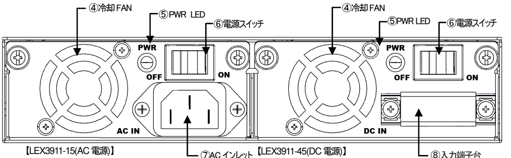
LEX3004 背面のイメージ図(LEX3911-45、LEX3911-15:1台搭載の場合)
