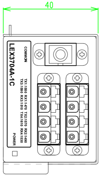
LEX3704A-1C
