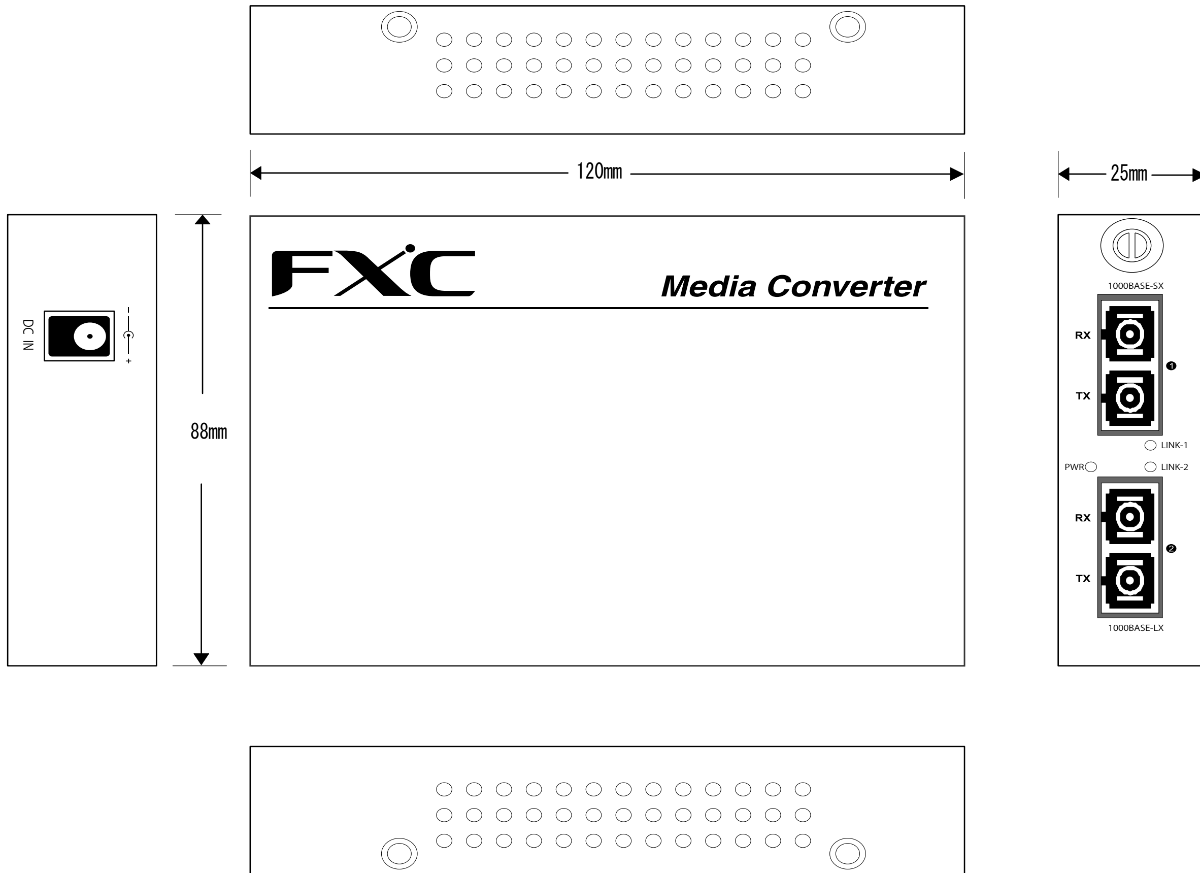
MC1100シリーズ外観図
