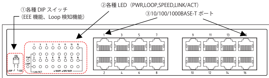
【前面図】
